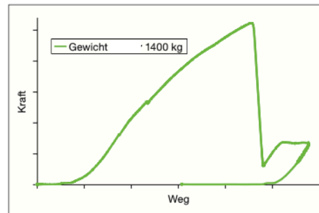
Bild 5: Darstellung des Zugkraft-Wegverlaufes
