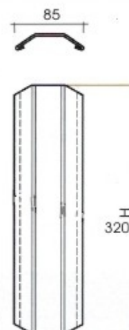
art. 44146 TRAVERSINO H 400 CENHTRALE
