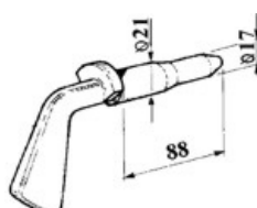
art. 25318 SPINOTTO D. 17/21 LUNGO gr. 430
