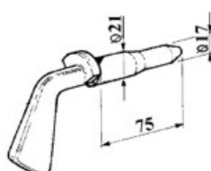
art. 25308 SPINOTTO D. 17/21 CORTO gr. 390
