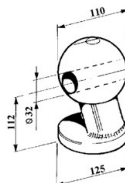
art. 25294 SFERA CON FORO D.110 gr. 7.910
