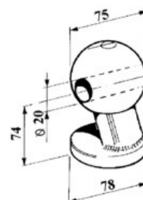
art. 25178 SFERA CON FORO D.75 gr. 2.320
