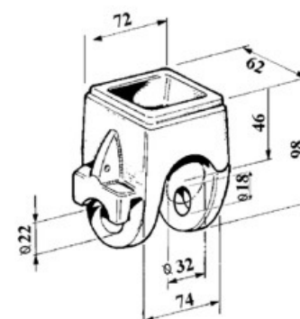
art. 25316 BOCCA DI LUPO FORI DIFFERENZIATI gr. 1.600
