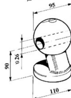
art. 25266 SFERA CON FORO D.95 gr. 4.780
