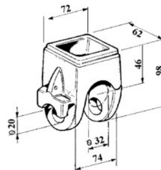
art. 25314 BOCCA DI LUPO gr. 1.600
