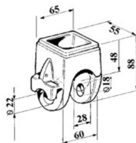
art. 25306 BOCCA DI LUPO FORI DIFFERENZIATI gr. 1.200
