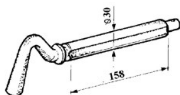
art. 25152 SPINOTTO D.30 1S gr. 1.230
