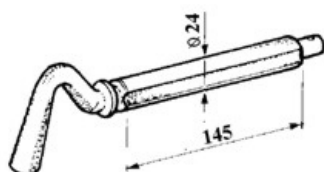
art. 25148 SPINOTTO D.24 1S gr. 770
