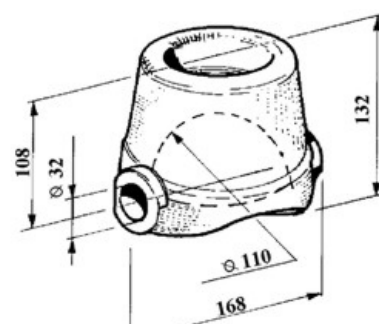
art. 25290 SUPPORTO SFERA D.110 gr. 9.450
