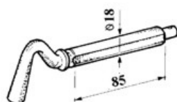
art. 25135 SPINOTTO D.18 1S CORTO gr. 310
