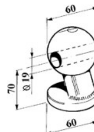
art. 25166 SFERA CON FORO D.60 gr. 1.340
