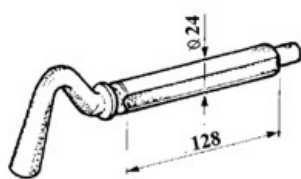
art. 25142 SPINOTTO D.24 1S gr. 720
