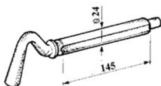
art. 25150 SPINOTTO D.24 2S gr. 770
