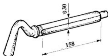
art. 25156 SPINOTTO D.30 2S gr. 1.230
