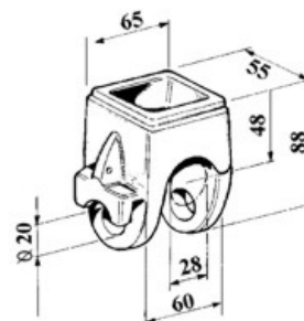
art. 25304 BOCCA DI LUPO gr. 1.200
