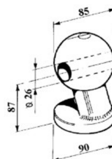
art. 25222 SFERA CON FORO D.85 gr. 3.370
