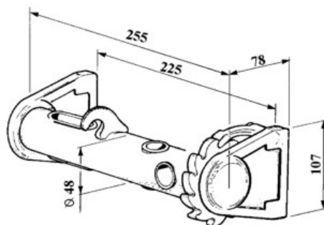
art. 30208 VERRICELLO D. 48 SUPP. STAMPATI C/TENDINASTRO gr. 3.000
