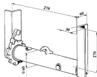
art. 30130 VERRICELLO D. 60 STAFFE L. 270 C/TUBINO gr. 3.900
