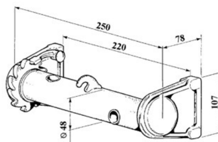
art. 30108 VERRICELLO D. 48 SUPP. STAMPATI C/TUBINO gr. 2.900
