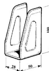
art. 46150 SUPPORTO ASTA CENTINA gr. 135
