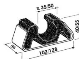
art. 46157 SUPP.GOMMA TUBO D.50 gr. 350
