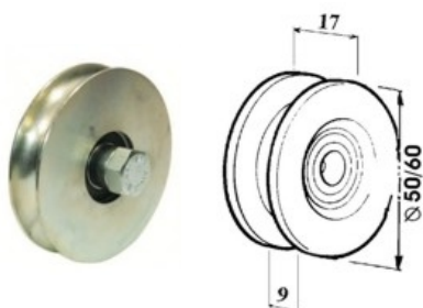
art. 46220 RUOTA ZINC.C/CUSC. DISTANZ.-BULLONE gr. 210 D.50 PORTATA Kg.100
