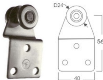
art. 46272 CARRELLO ZINC.2 CUSC. SAG. gr. 80 PORTATA Kg. 40
