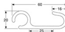
art. 46742 BARRA T.TELONE IN ALLUMINIO L. 3250
