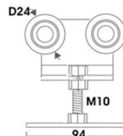
art. 46340 CARRELLO ZINC. 4 CUSCINETTI C/PIASTRA E BULLONE gr. 260 PORTATA Kg. 50
