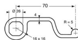
art. 46730 PROFILO DI TENSIONE IN ALLUMINIO L. 3250
