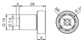
art. 46816 CUSCINETTO SESAM gr. 200
