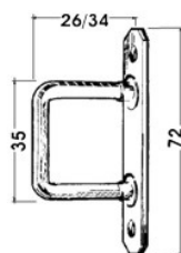
art. 46142 ANELLO TELONE QUADRO H26 gr. 35
