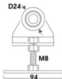
art. 46320 CARRELLO ZINC. 2 CUSCINETTI C/PIASTRA E BULLONE gr. 190 PORTATA Kg. 40
