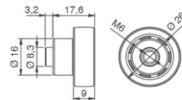
art. 46820 CUSCINETTO ROSSO VERSUS gr. 100
