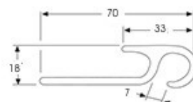
art. 46744 BARRA T.TELONE IN ALLUMINIO L. 3250
