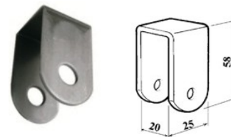
art. 46222 SUPPORTO PER RUOTA gr. 110
