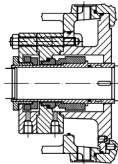
Tenuta meccanica doppia Double mechanical seal
