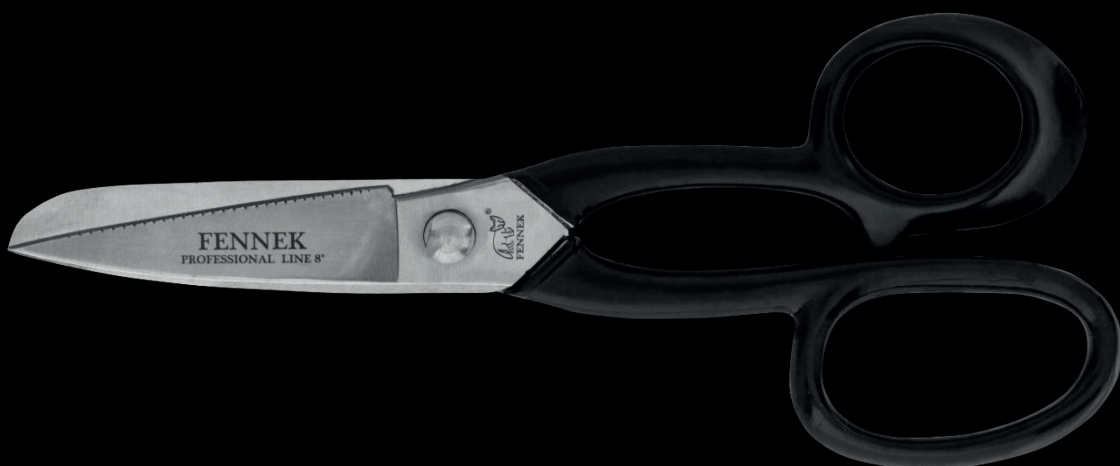
Art. 157 CESOIA PER CUOIO manici verniciati - lame brunite poll. 8 - 10 LEATHER CUTTING SHEARS black handles - satin blades
