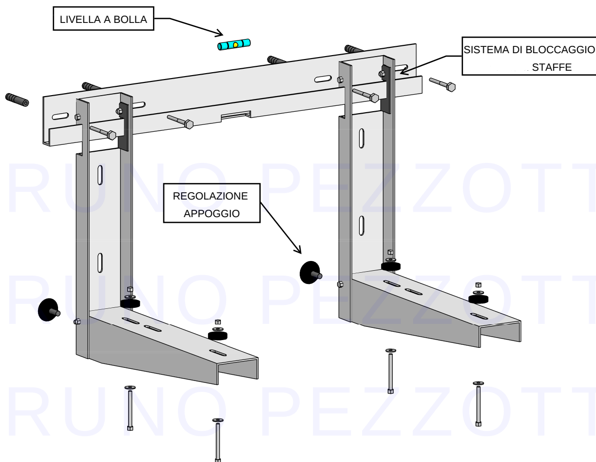
ASSONOMETRIA MONTAGGIO STAFFE AXONOMETRY MOUNTING BRACKETS
