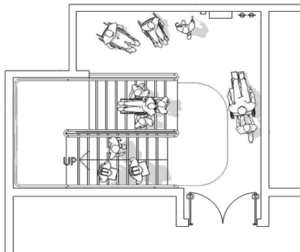
Illustrazione S.4-5: Esempio di spazio calmo (area of rescue assistance) secondo ISO 21542
