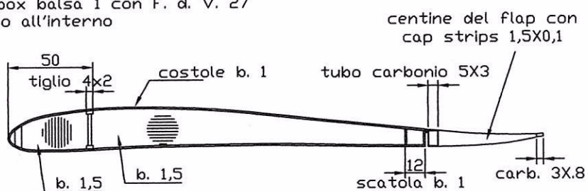
Sezione tipo parte centrale Profilo T5
