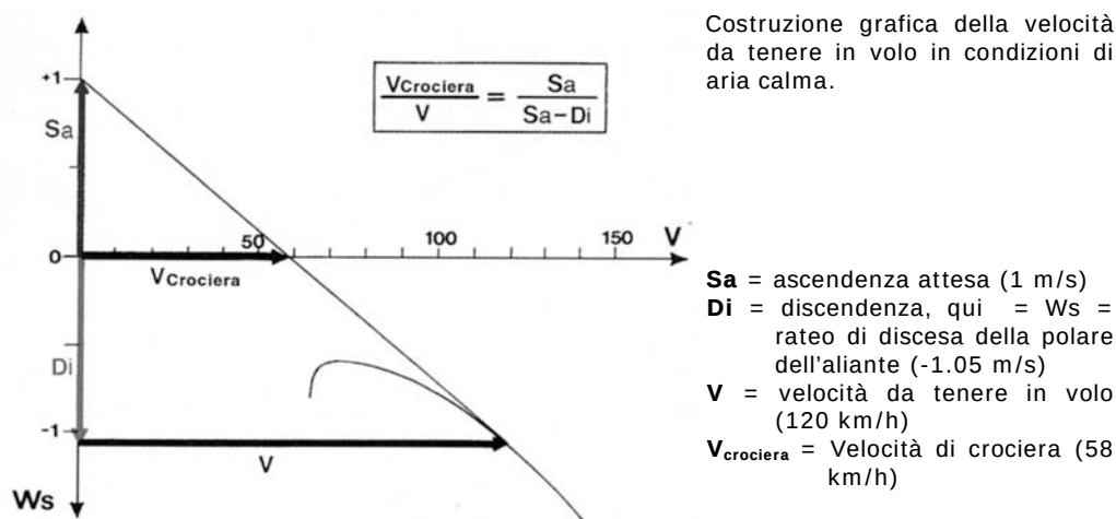
DETERMINAZIONE GRAFICA DELLA VELOCITÀ DA TENERE IN ARIA CALMA
