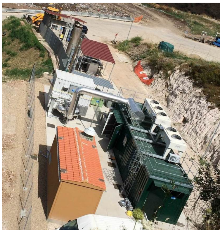
Figura 5: Impianto produzione energia elettrica – Vista dall'alto
