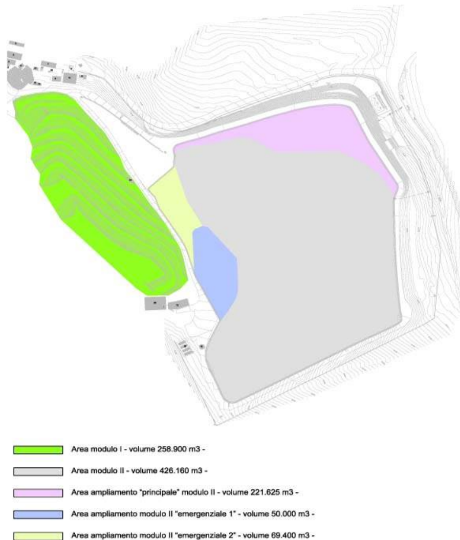
Figura 4: Planimetria impianto – indicazione moduli discarica
