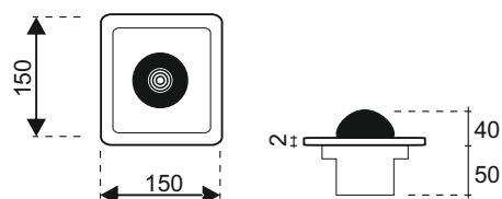
I 30 PA 001 Comando pneumatico inox a pedale per il montaggio a pavimento completo di tubo corrugato di mt. 2
