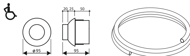
Comando pneu nova in ABS bianco incasso completo di tubo corrugato di mt. 2
