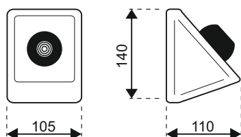
I 30 PA 000 Comando pneumatico inox a parete e/o a pavimento completo di tubo corrugato di mt. 2
