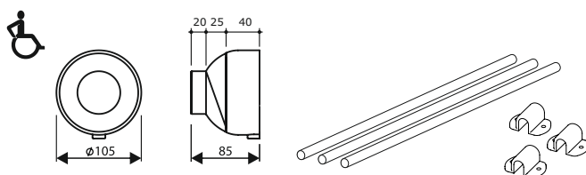
Comando pneu nova in ABS bianco, esterno a parete completo di accessori per fissaggio
