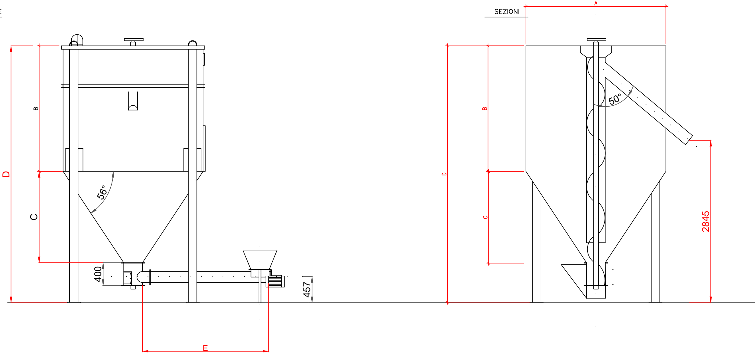
VISTA LATERALE
