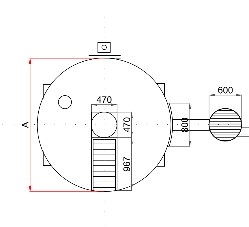
VISTA DALL'ALTO
