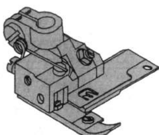
257321A64 Piedino * 3 Aghi
