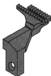
257293-16F Griffa anteriore
