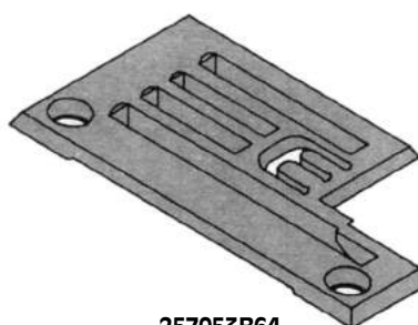
257053B64 Placca ago
