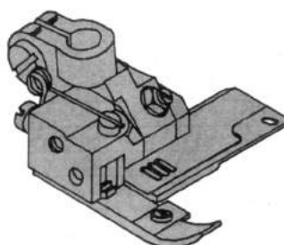
257326A64 Piedino * 3 Aghi
