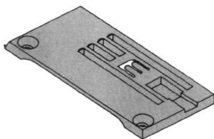
14-8630 Placca ago
