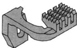
15-7230-0 Griffa anteriore
