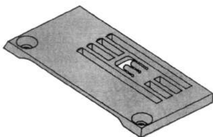
14-8640-0 Placca ago
