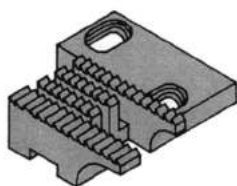
15-8280-0 Griffa posteriore
