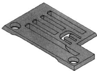
14-8660-0 Placca ago
