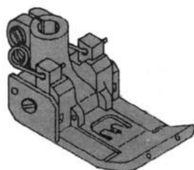
0064042 Piedino
