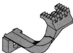
15-9070-0 Griffa posteriore
