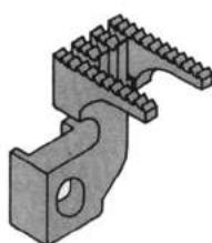
15-9070-0 Griffa posteriore
