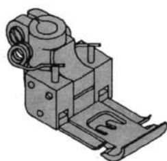
17-8940-1 Piedino
