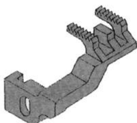
9109030 Griffa anteriore
