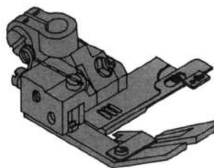
257326A64 Piedino
