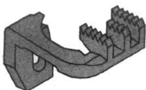
15-7610-0 Griffa anteriore
