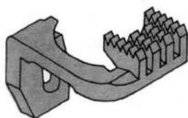
15-7530-0 Griffa posteriore
