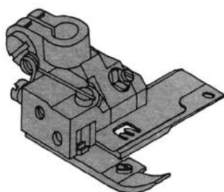
257421-64 Piedino
