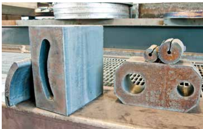
Esempi di taglio • Cutting examples
