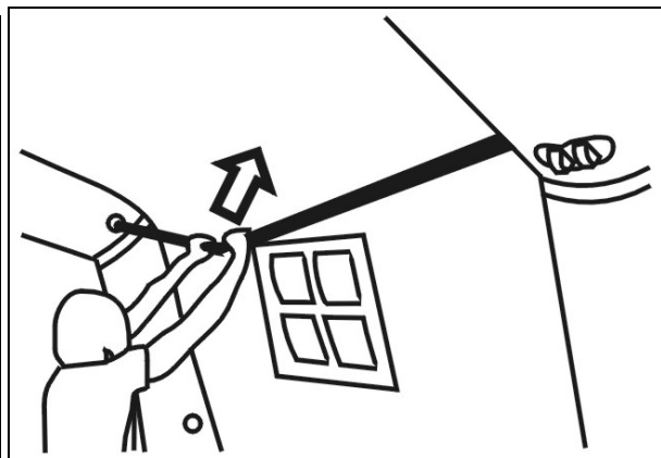
Figura 2.6 - Montaggio asta distanziale snodata.
