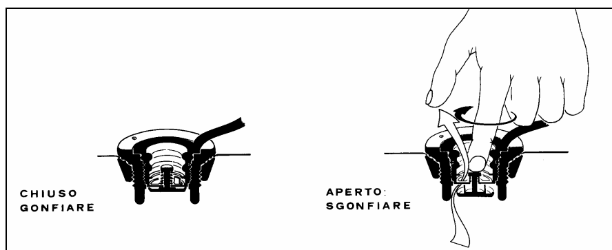
Figura 2.1 – Chiusura delle valvole di gonfiaggio.
