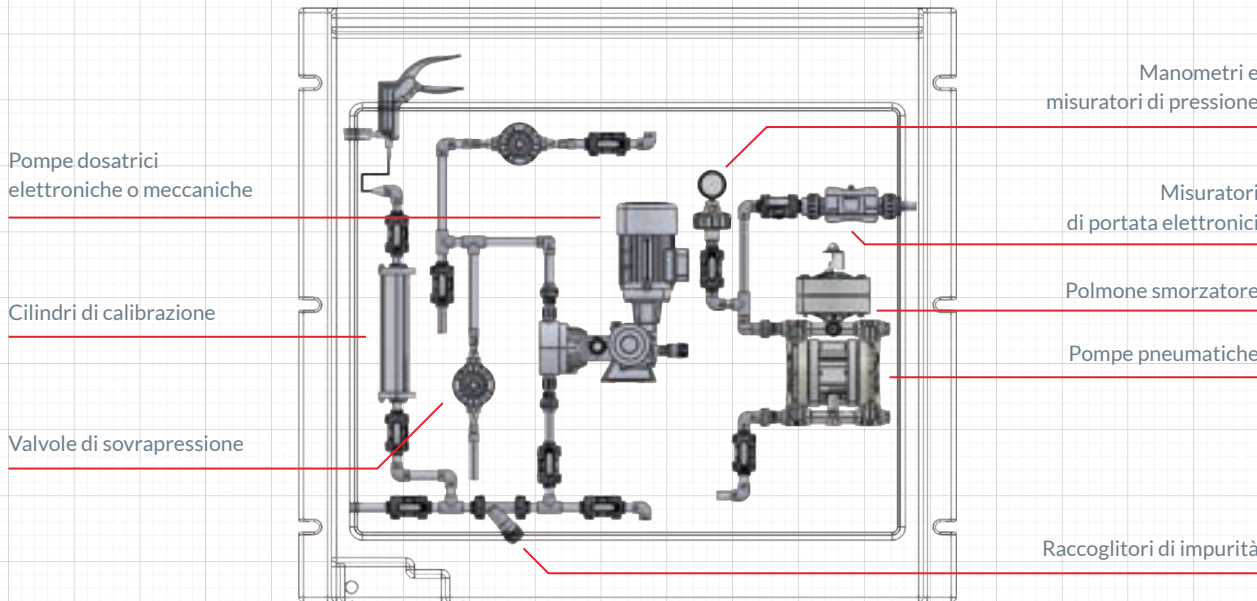
Schema
