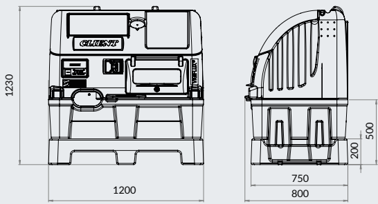
Dimensioni
