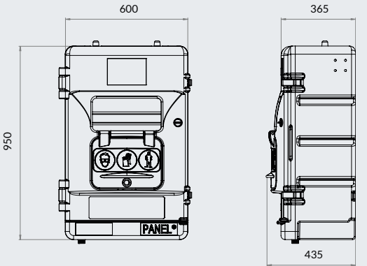
Dimensioni
