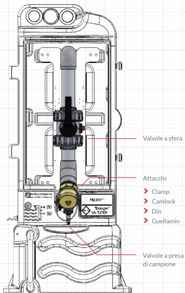
Schema
