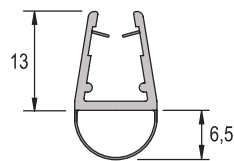
Guarnizione a palloncino Balloon gasket
