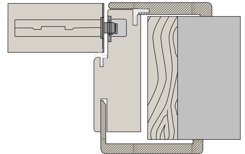
Restiling del telaio Restyling of the frame
