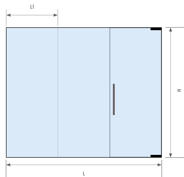
Soluzione con porta 1TV a bilico apribile Solution with pivoting 1TV door
