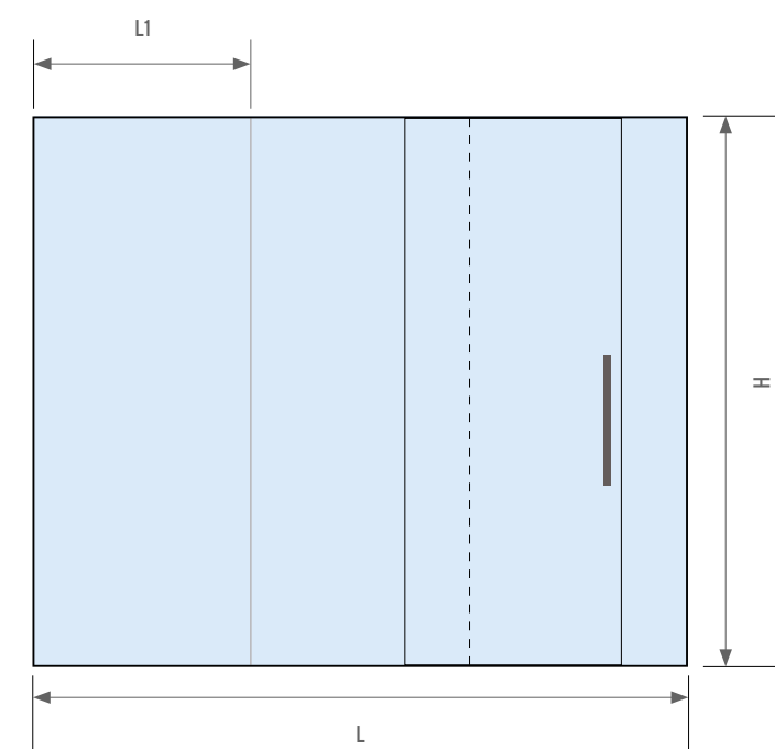
Soluzione con porta 1TV scorrevole Solution with sliding 1TV door
