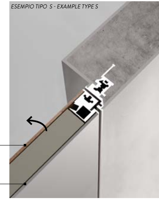
MURATURA - MASONRY ESEMPIO TIPO S - EXAMPLE TYPE S
