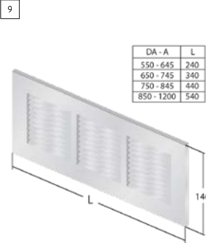
GRIGLIA PER AERAZIONE VENTILATION GRILLE IN METAL
