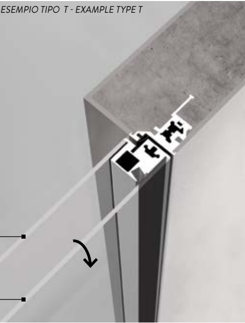
MURATURA - MASONRY ESEMPIO TIPO T - EXAMPLE TYPE T
