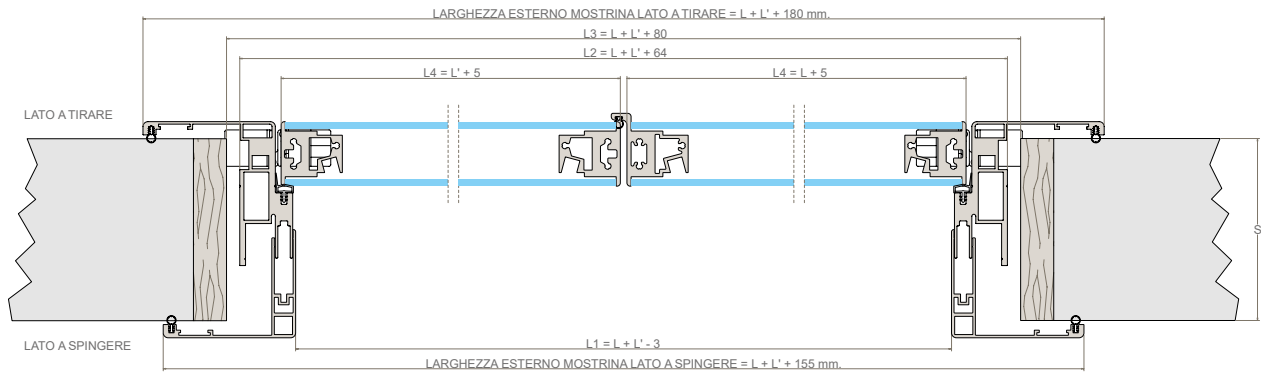
SEZIONE ORIZZONTALE
