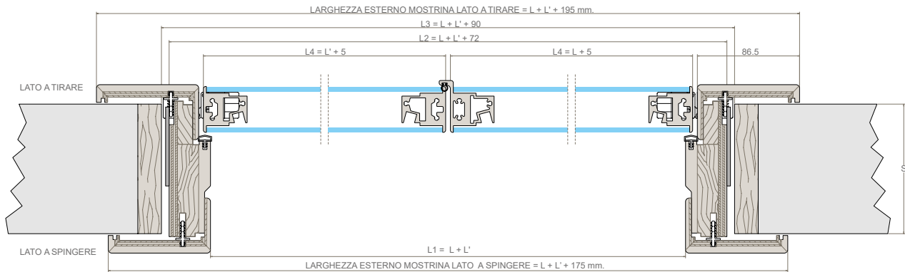
SEZIONE ORIZZONTALE
