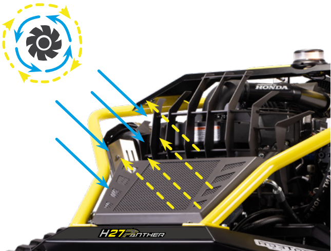
INVERSIONE VENTOLA DI RAFFREDDAMENTO per pulizia radiatore INVERSION OF COOLING FAN MOTION for cleaning the radiator
