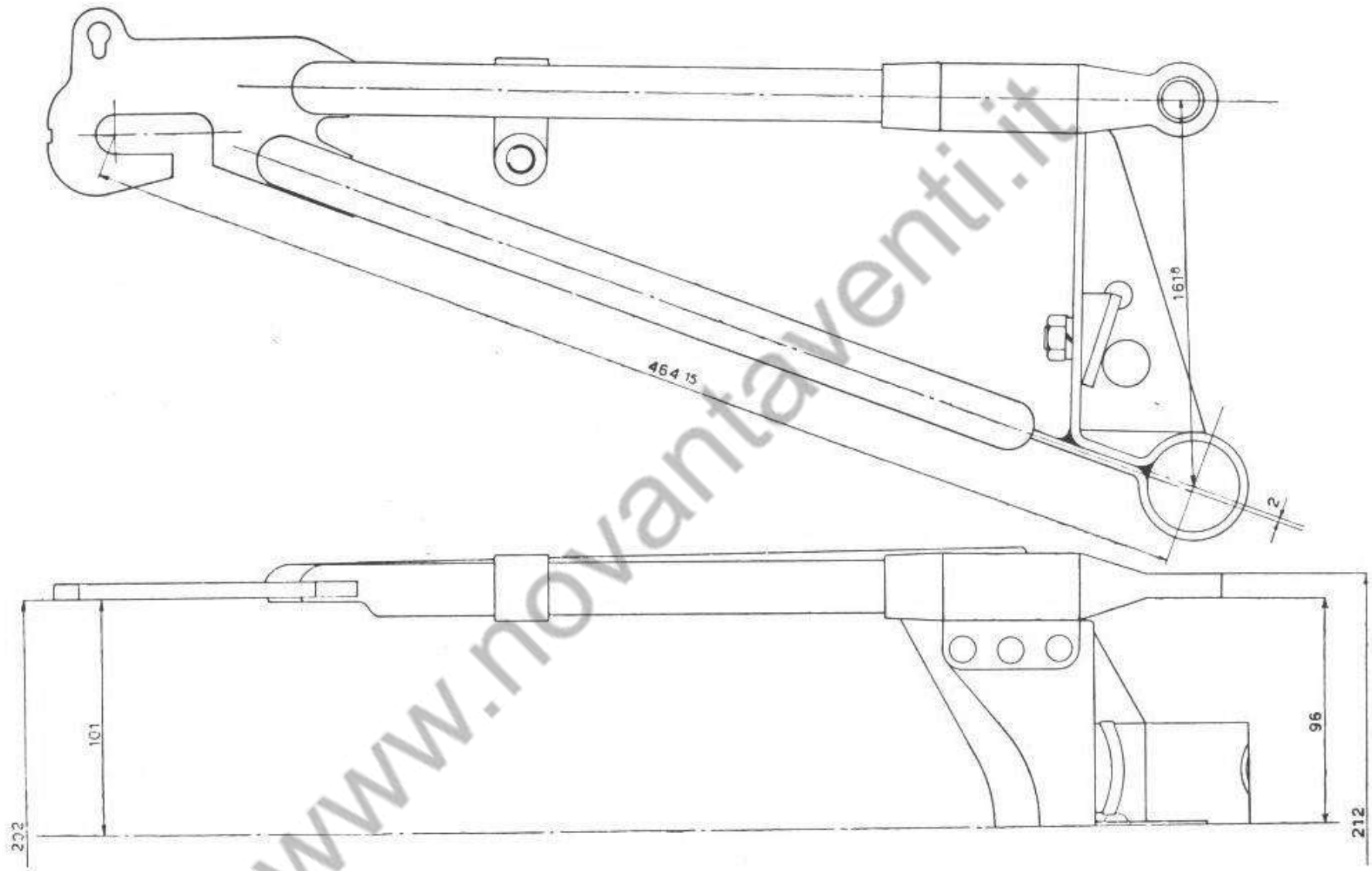
Fig. 35 - Forcellone oscillante
