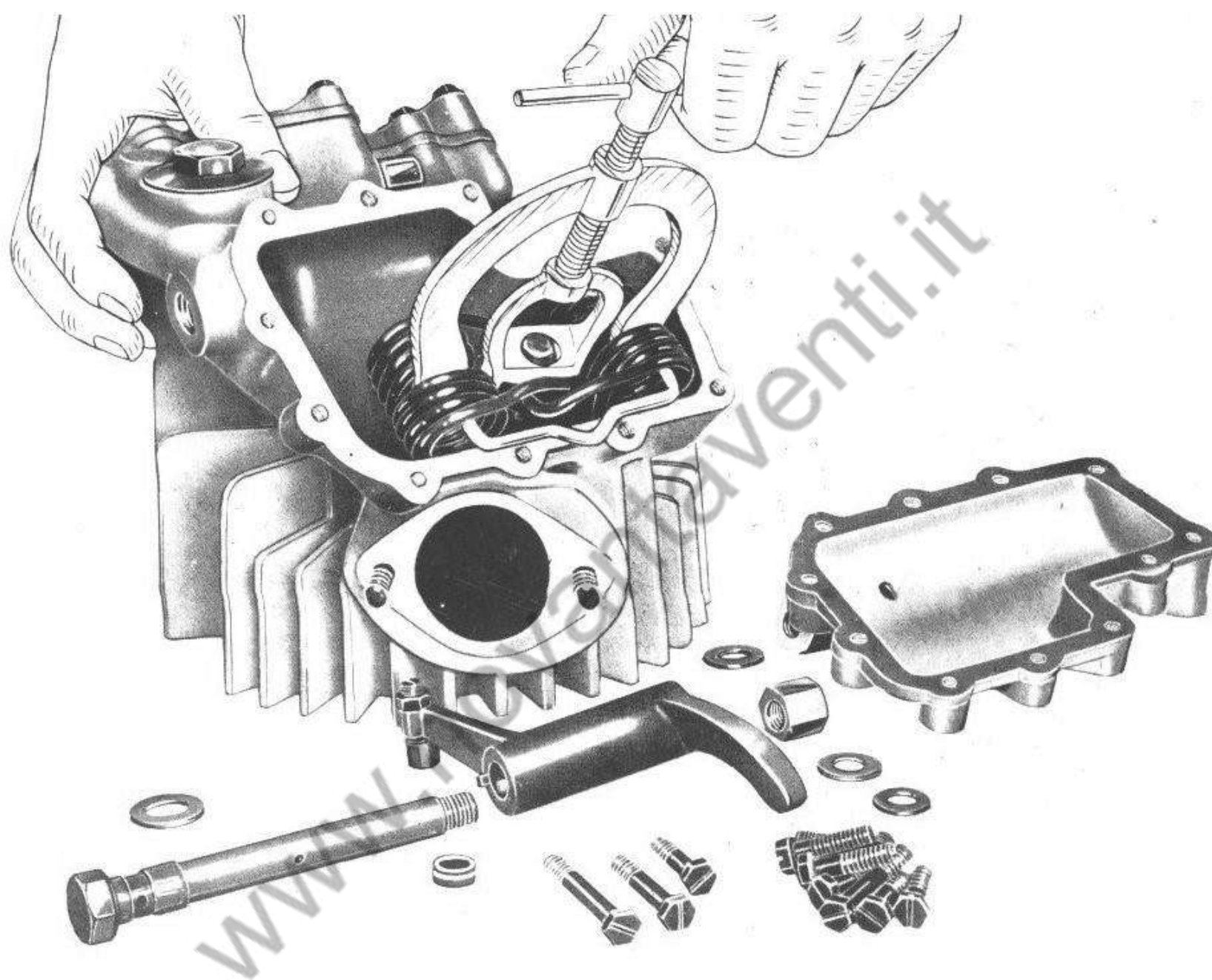
Fig. 19 - Come viene eseguita l'estrazione delle molle dalla testa
