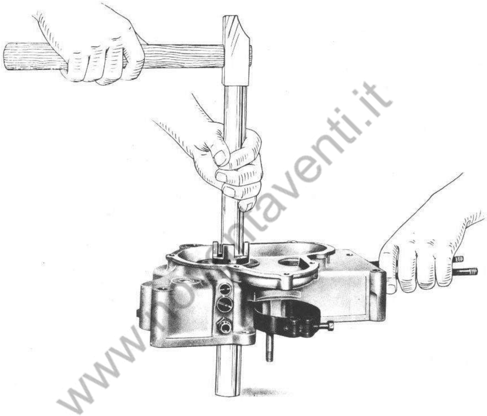
Fig. 16 - Come si sfila l'albero primario del cambio
