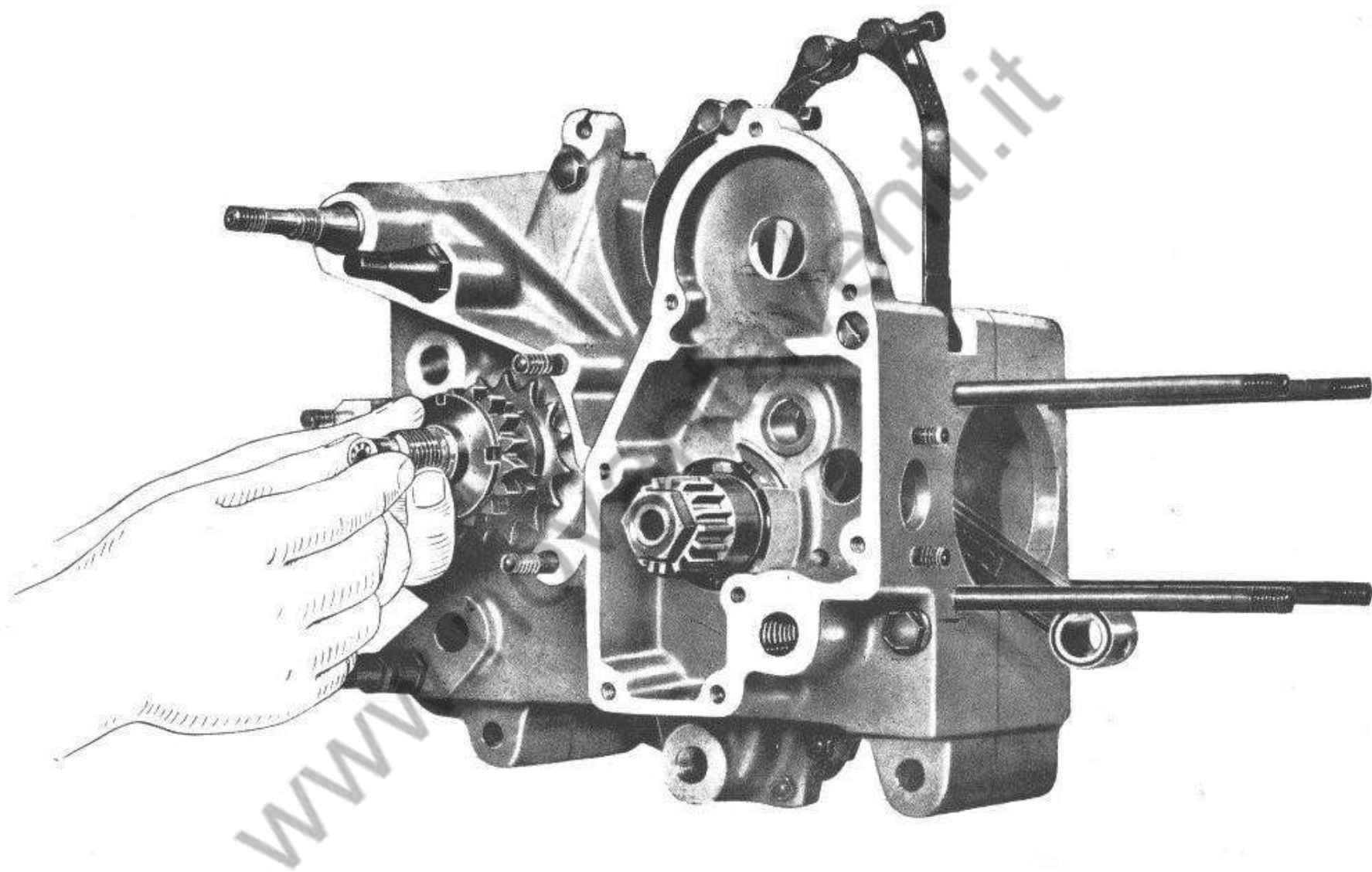
Fig. 10 - Come si smonta l'asta di comando frizione
